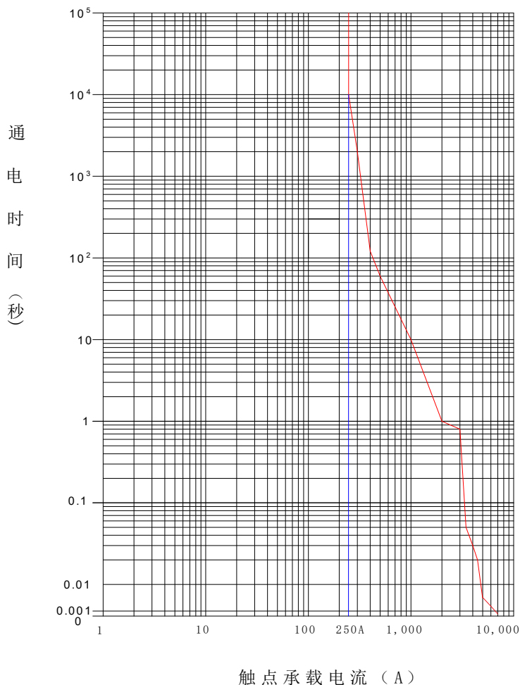
EVL250 通电性能曲线 (85℃时) (不爆炸、不起火)
